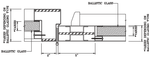
DOOR JAMB AT HINGE
