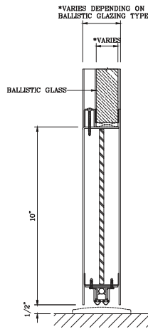
DOOR BOTTOM RAIL DETAIL
