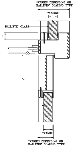
DOOR TOP RAIL DETAIL
