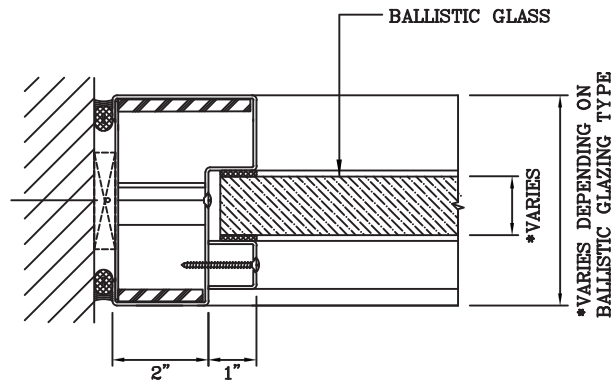
1 JAMB DETAIL
