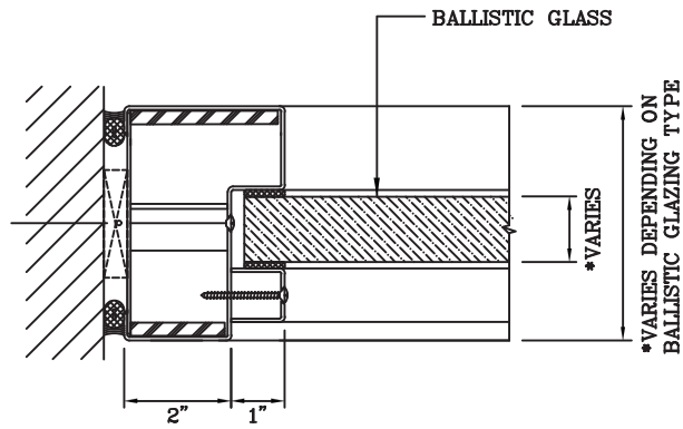
1 JAMB DETAIL
