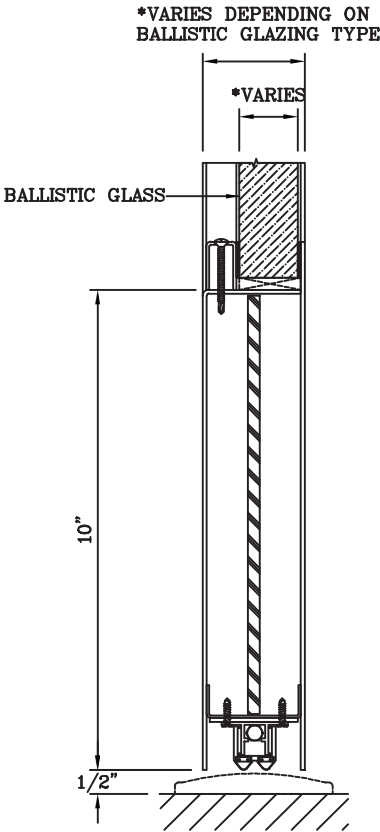
1 - DOOR BOTTOM RAIL DETAIL
